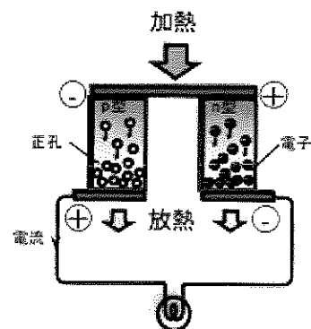
図 1 熱電発電の原理
