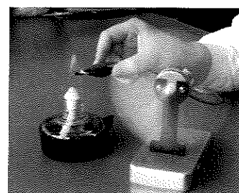
図 2 熱電発電素子による発電のデモ
