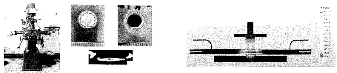
摩擦攪拌接合
