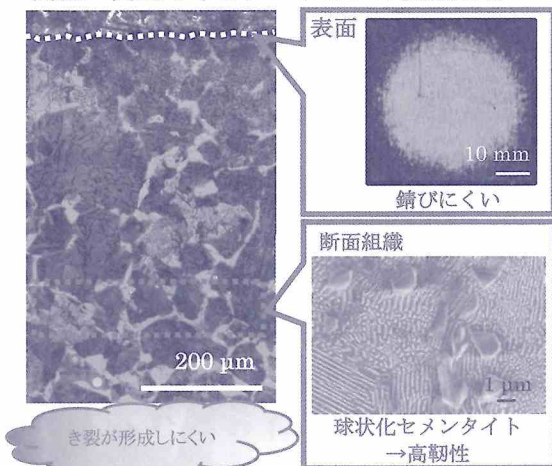
図2 鉄表面の高温高压気泡の加工
