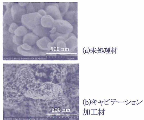
図3 光触媒酸化チタン粉末の高温高压気泡の加工
