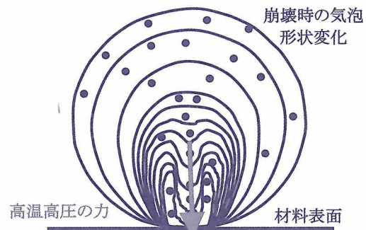
図1 気泡崩壊時の高温(数万℃)、高压(数万気圧)の力で表面を加工
