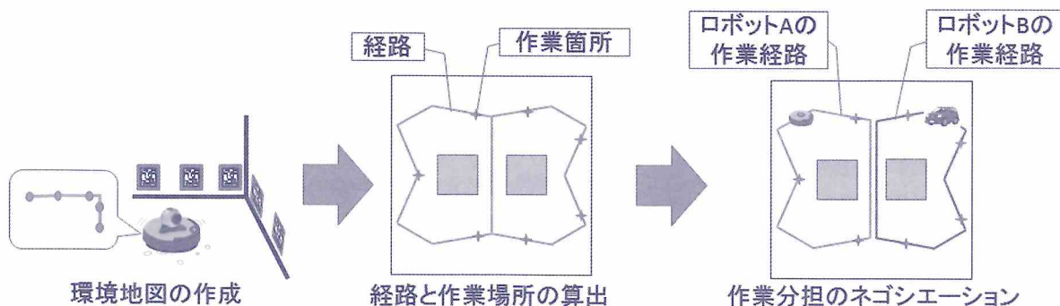
図1 自律ロボットシステムの動作概要
