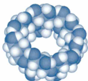
図1 シクロデキストリンの分子モデル
