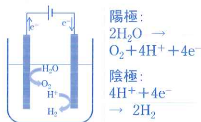
(a) 通常金属電極を使用
