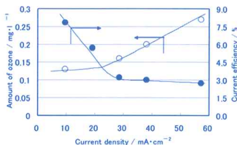
図 3 生成効率の電流密度依存性
