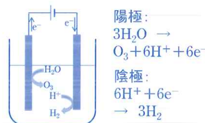
(b) 酸化電極を使用
