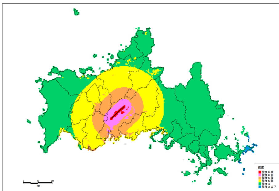
図4 大原湖断層系（山口盆地北西縁断層）
