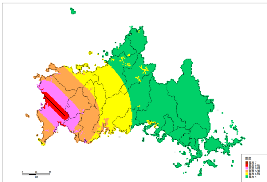
図2 菊川断層
